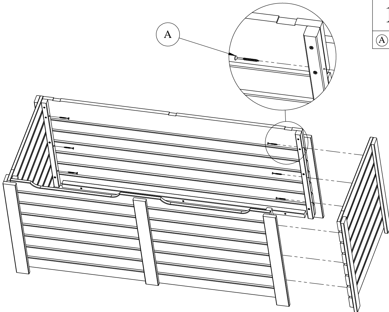
A - Ø4 x 45 - 12
